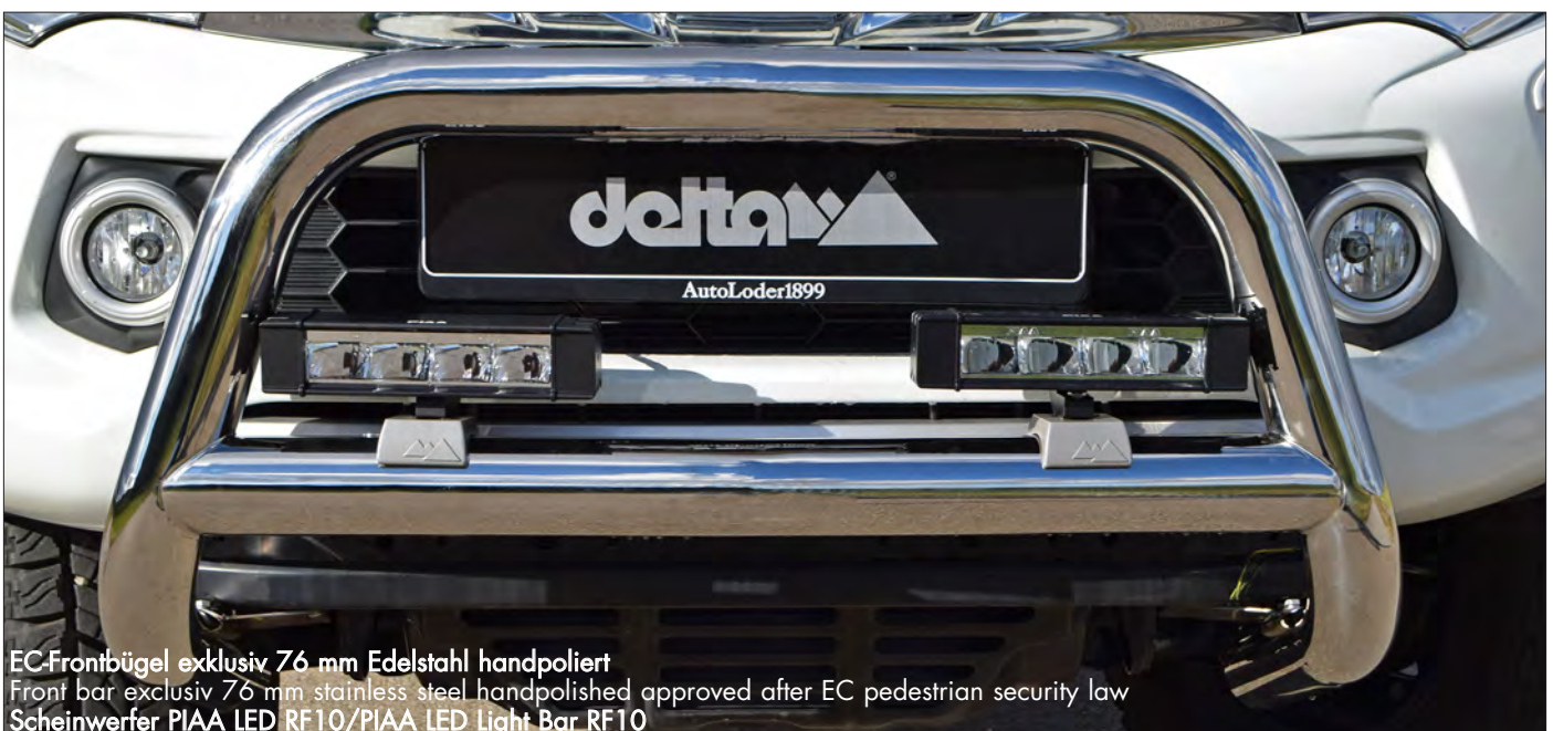
EC-Frontbügel exklusiv 76 mm Edelstahl handpoliert mit Unterfahrschutz Front bar exklusiv 76 mm stainless steel handpolished approved after EC pedestrian security law with Under Ride protection Scheinwerfer LED PIAA 570 und Anbausatz/Lights LED PIAA 570 and brackets basic
